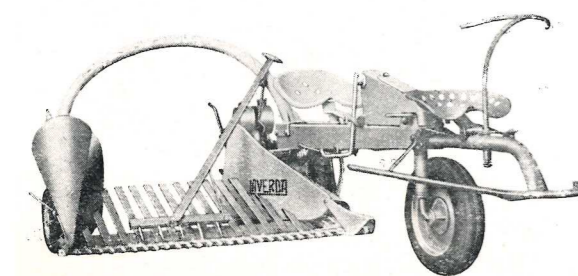
Motofalciatrice MF 4 L con apparecchio a mietero
