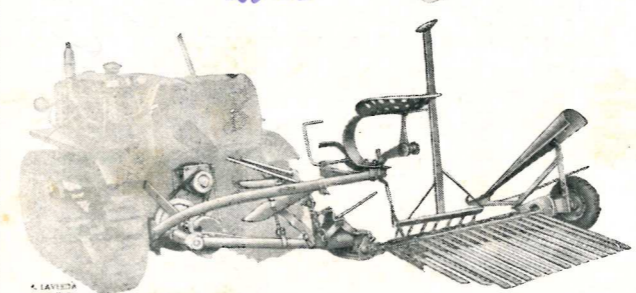
Apparecchio a mietere per "FAP 51,"
