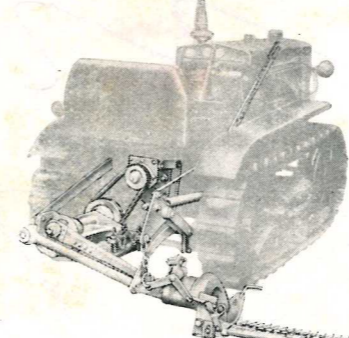
Falciatrice portata laterale "FAL 25 R,"
