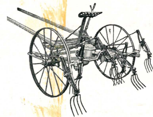
Voltafieno a forche mod. "VF 6 BO.,
