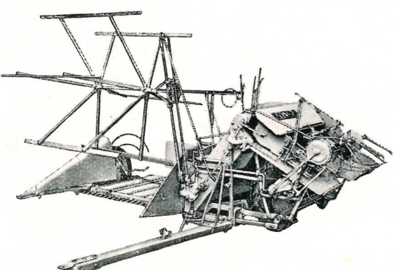
Mietitrice - Legatrice mod. "ML 6,"
