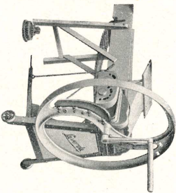
TRINCIAFORAGGIO Mod. FI
