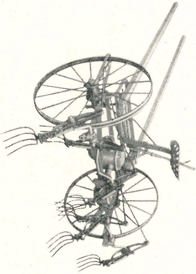
VOLTAFFIENO A FORCHE Mod. VF 6 80
