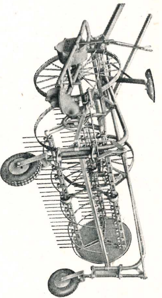
RANGHINATORE - VOLTAFIENO RV 6 BO
