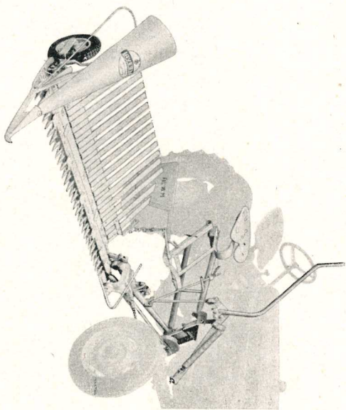
FALCIATRICE PORTATA LATERALE « FAL 18 M » CON APPARECCHIO A MIETERE, MONTATO
