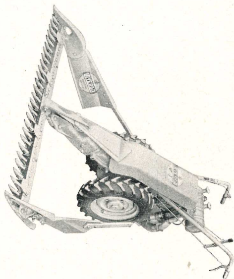
MOTOFALCIATRICE Mod. MF 4
