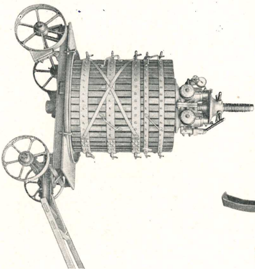
CARRELLO A 4 RUOTE PER TORCHI
