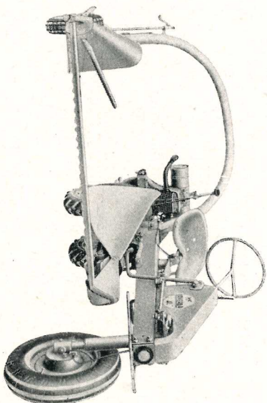
MOTOFALCIATRICE Mod. MF 4 L
