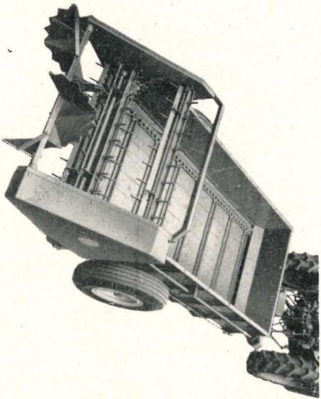
RIMORCHIO SPANDILETAME COMBINATO Mod. RSC 3
