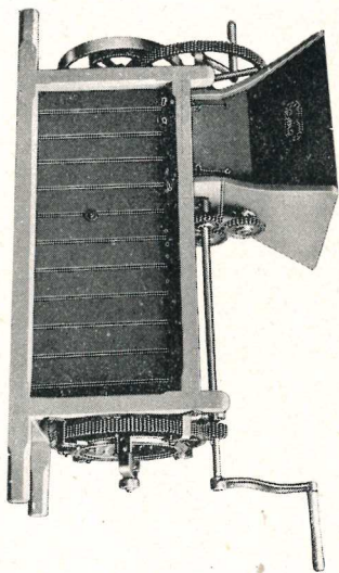
PIGIATRICE - DIRASPATRICE A TAMBURO ROTANTE
